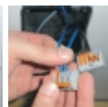
Leitungen abisolieren und in die Quick-Verbinder stecken (blau zu blau, schwarz zu schwarz). Quick-Verbinder schließen, so werden alle Matten parallel miteinander verbunden.
