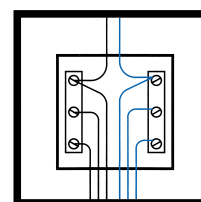
Jetzt noch eine Hin- und eine Rückleitung zum Regler einsetzen, schon können die Heizmatten in Betrieb genommen werden
